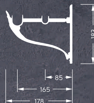
Лавр Ø28/19
