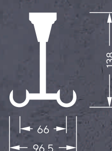
потолочный Ø19/19
