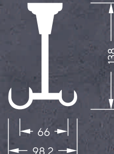
потолочный Ø25/16
