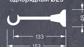
однорядный Ø25
