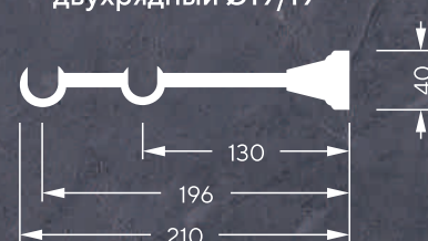
двухрядный Ø19/19
