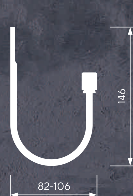
Захват Ø16
